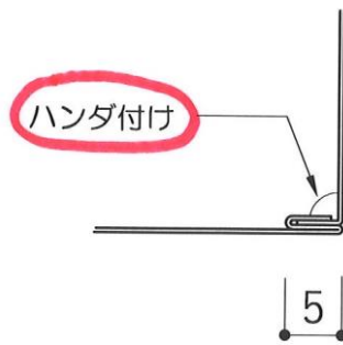
[D-D'詳細図]
