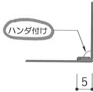
[D-D'詳細図]
